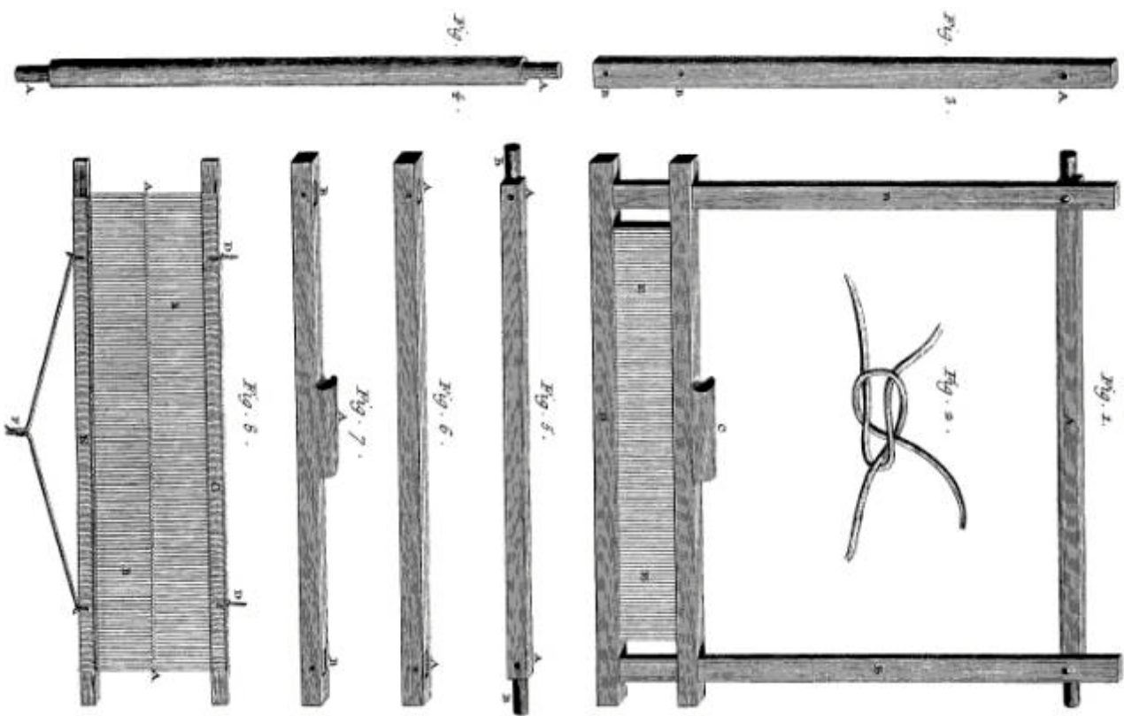
Tisserand, Détails du Mécanisme à faire la Toile.
